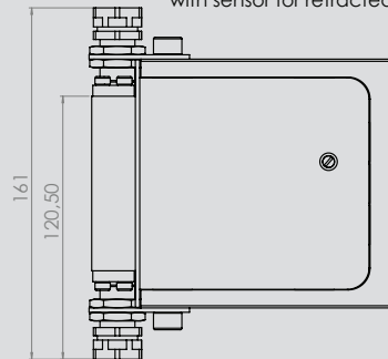
mit Abfrage Anschlag eingefahren with sensor for retracted stop
