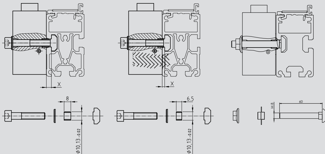
Befestigungssatz C Assembly kit C Heavy-Duty (No 44000667)
